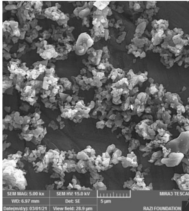
تصویر میکروسکوپی از ریز ساختار پودر آلفا آلومینا.
