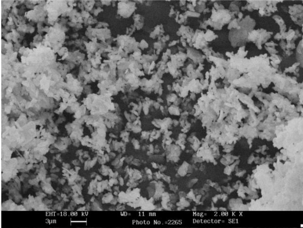
تصویر میکروسکوپی از ریز ساختار پودر آلفا آلومینا.
