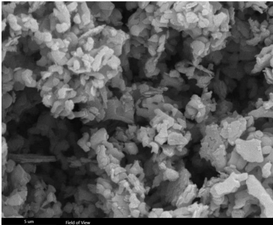
تصویر میکروسکوپی از ریز ساختار پودر آلفا آلومینا.
