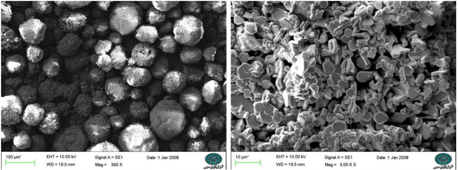
تصویر میکروسکوپی از ریز ساختار پودر آلفا آلومینا.
