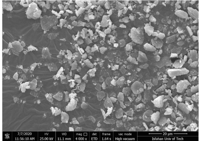
تصویر میکروسکوپی از ریز ساختار پودر آلفا آلومینا.
