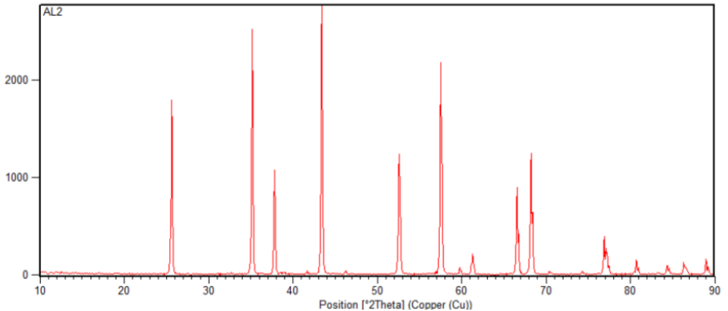
الگوی پراش پرتو ایکس از پودر آلفا آلومینا
